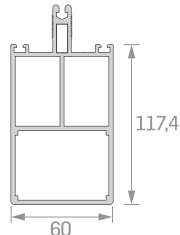
1653 Griyaj Profili GRIYAJ PROFILE Ağırlık / Weight: 2,724
