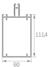
5770 Griyaj Profili GRIYAJ PROFILE Ağırlık / Weight: 1,799
