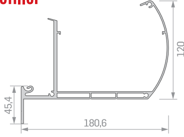
1656 Oluk Profili BORDER PROFILE Ağırlık / Weight: 4,046
