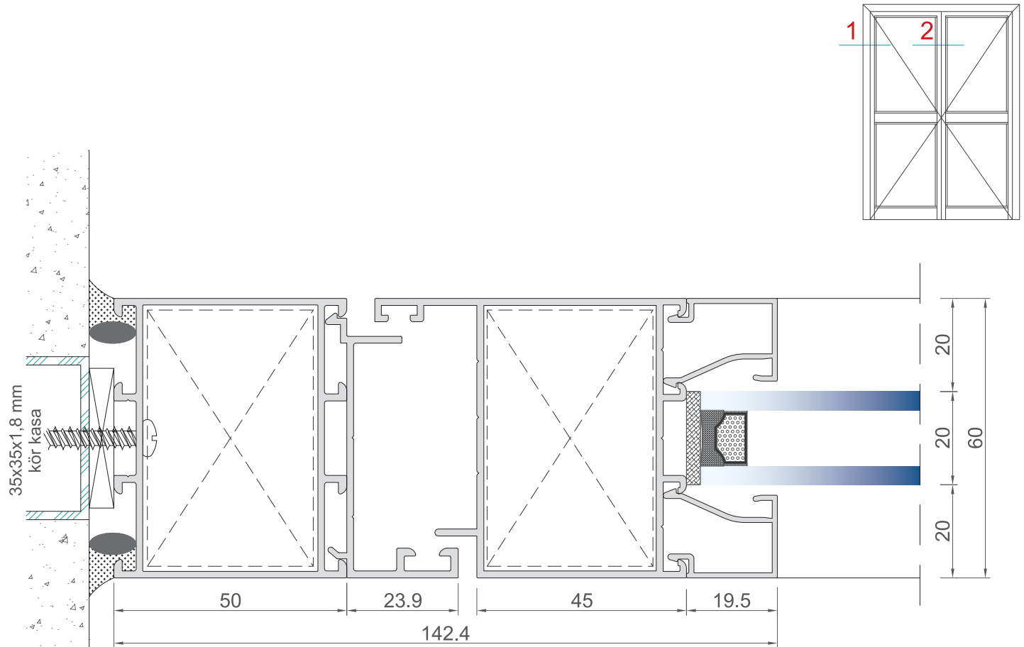
Kesit-1
