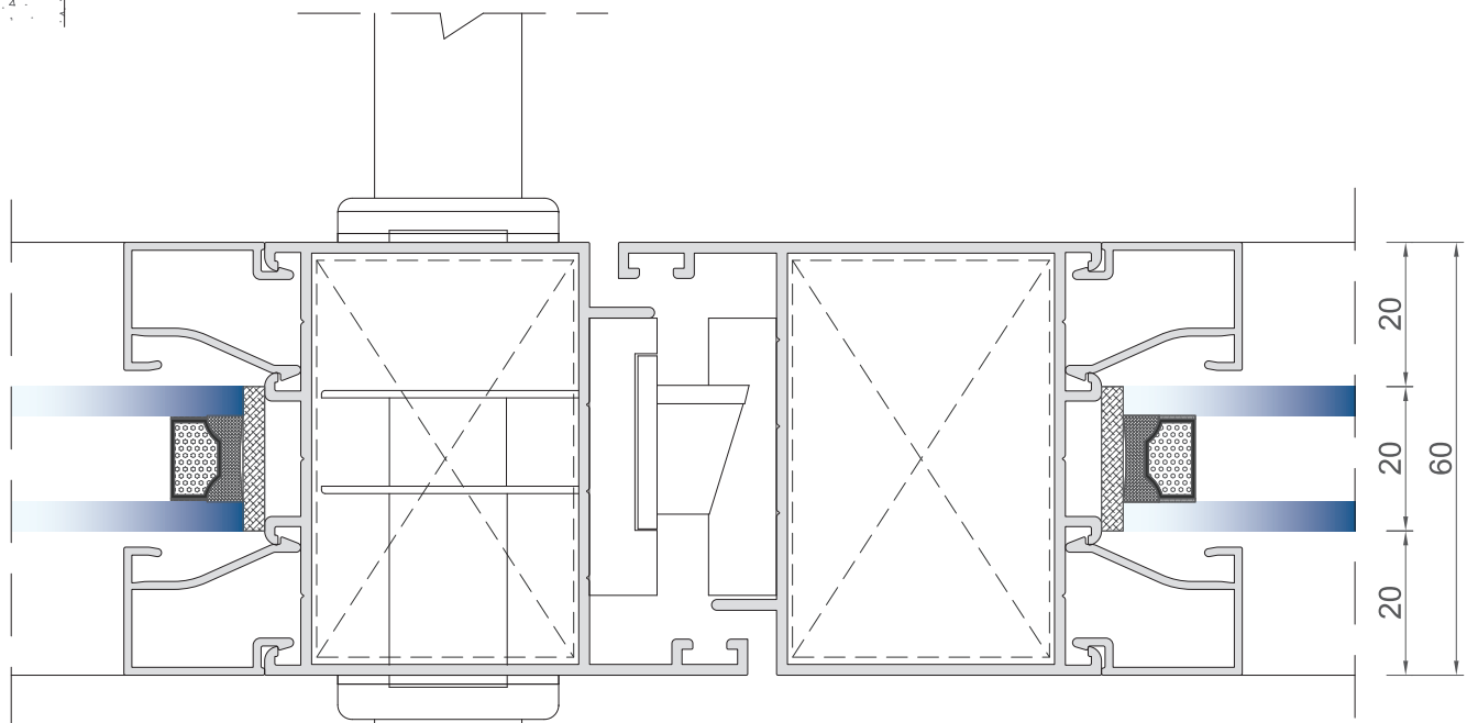
Kesit-2
