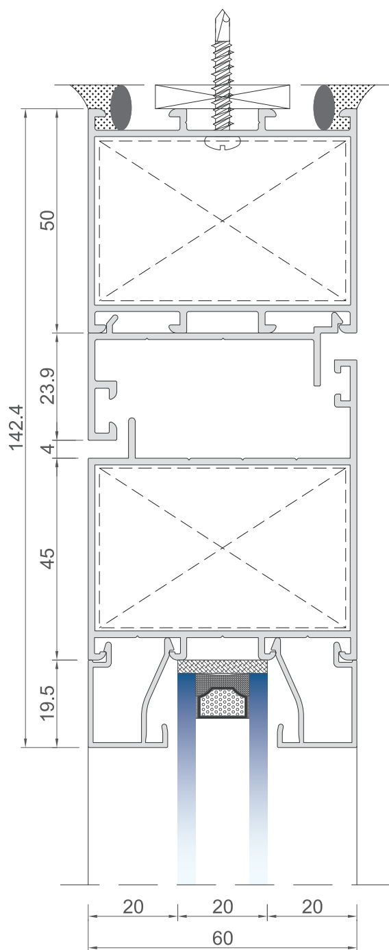
Kesit-3
