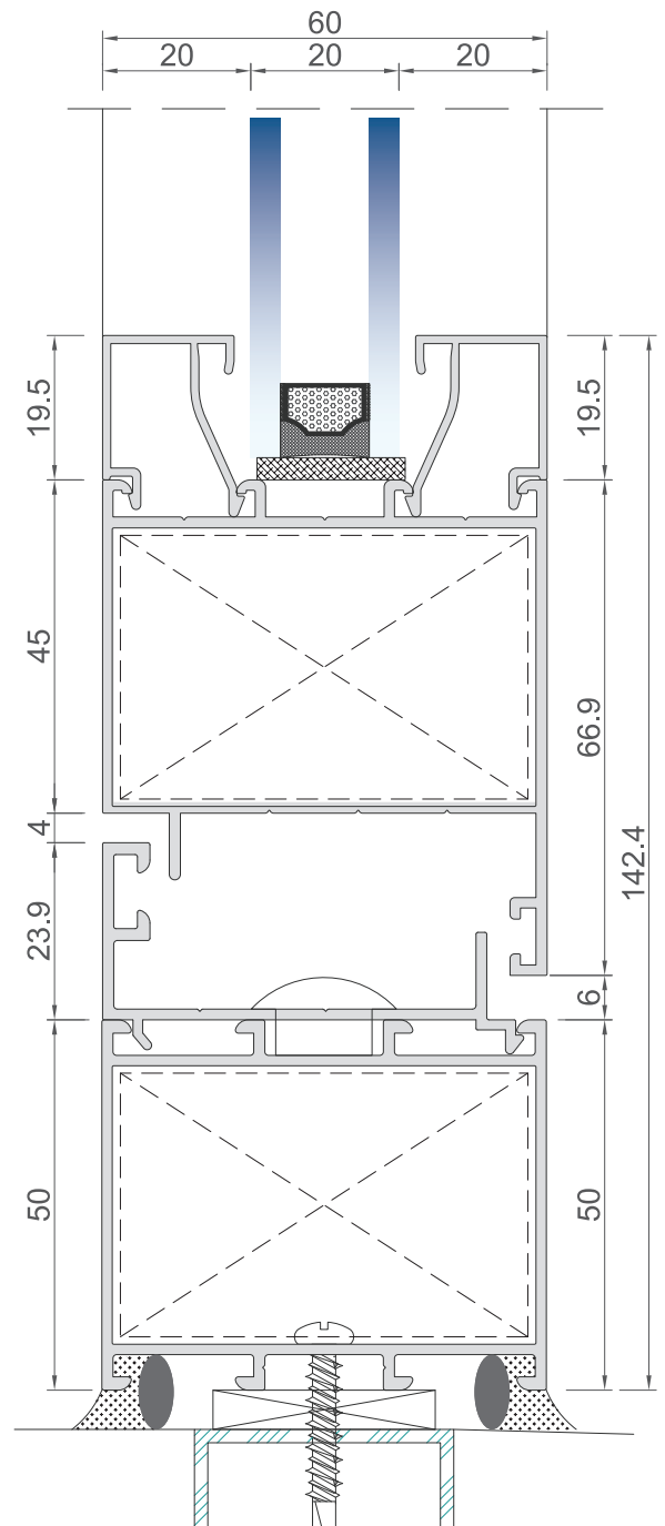
Kesit-7
