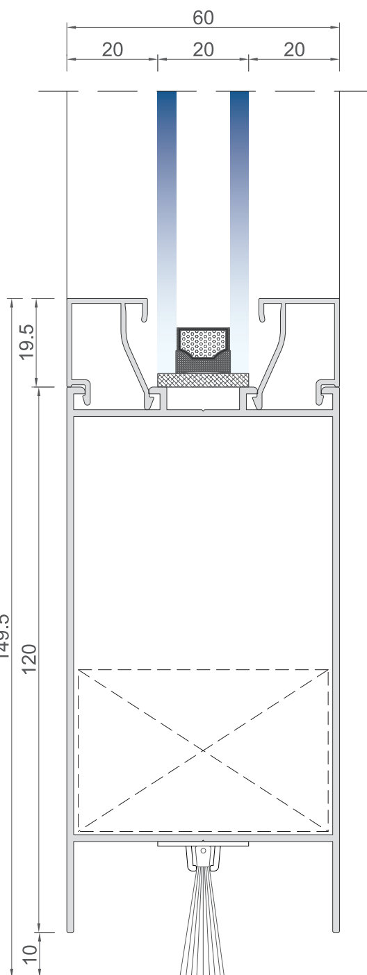
Kesit-4
