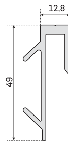
1676 - 0,577 kg/m
